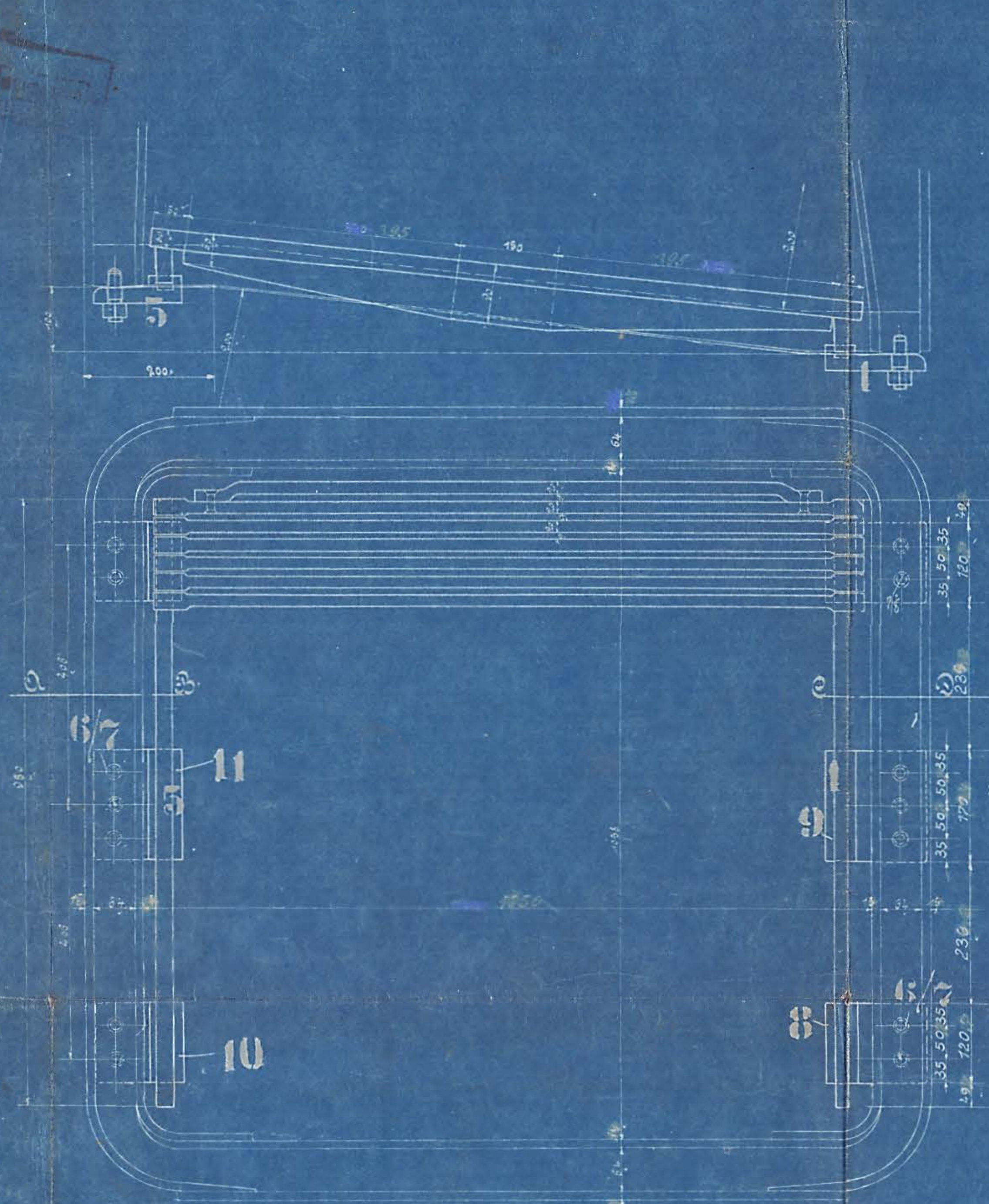
Schnitt A-B.
