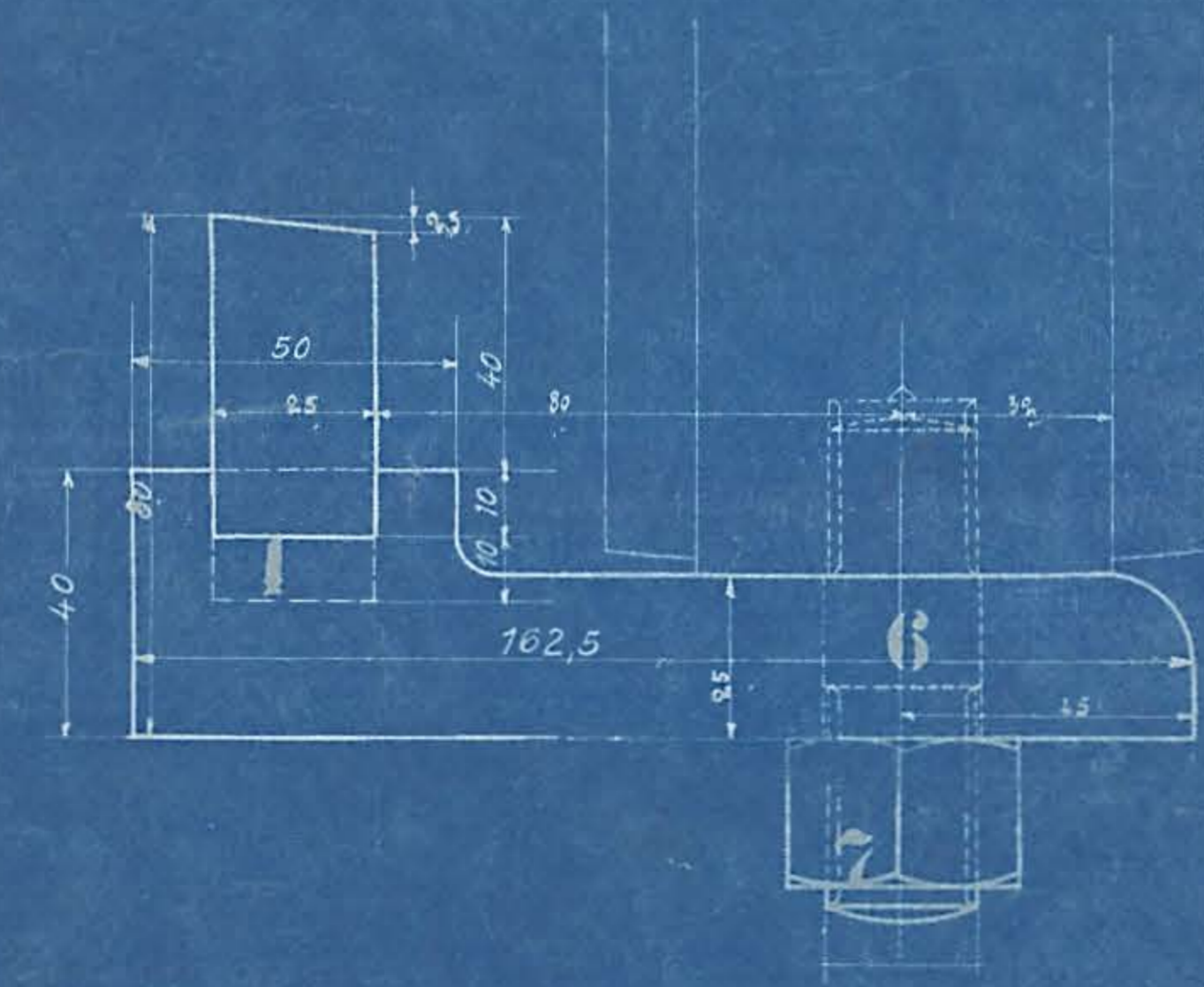
Schnitt C-D.
