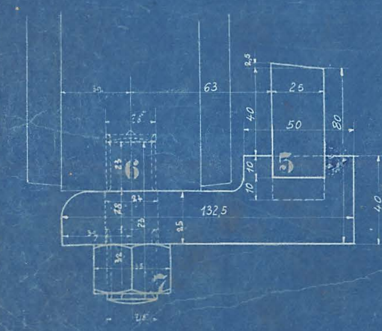
Schnitt A-B.
