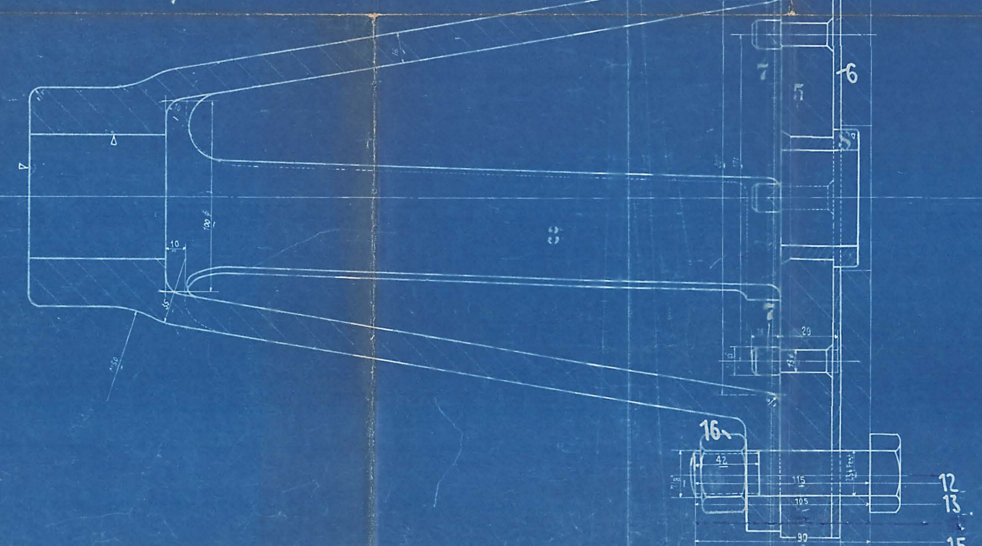
Schnitt A-B.
