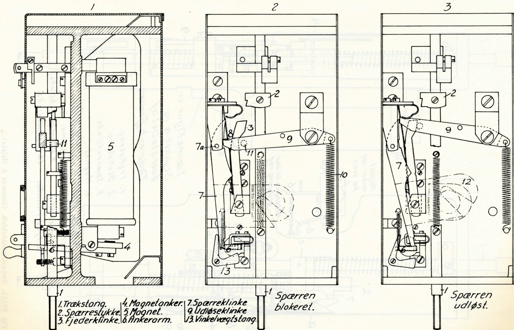
Fig. 0518b. Elektrisk trykknapspærre. (Siemens & Halske). Kontaktnordning er ikke medtaget i figuren.
