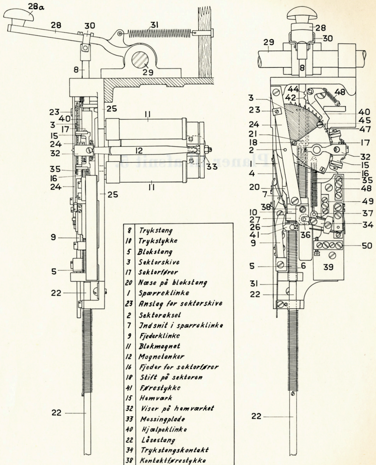
Fig. 0503b. Vekselstrømsblokfelt. (Siemens & Halske).
