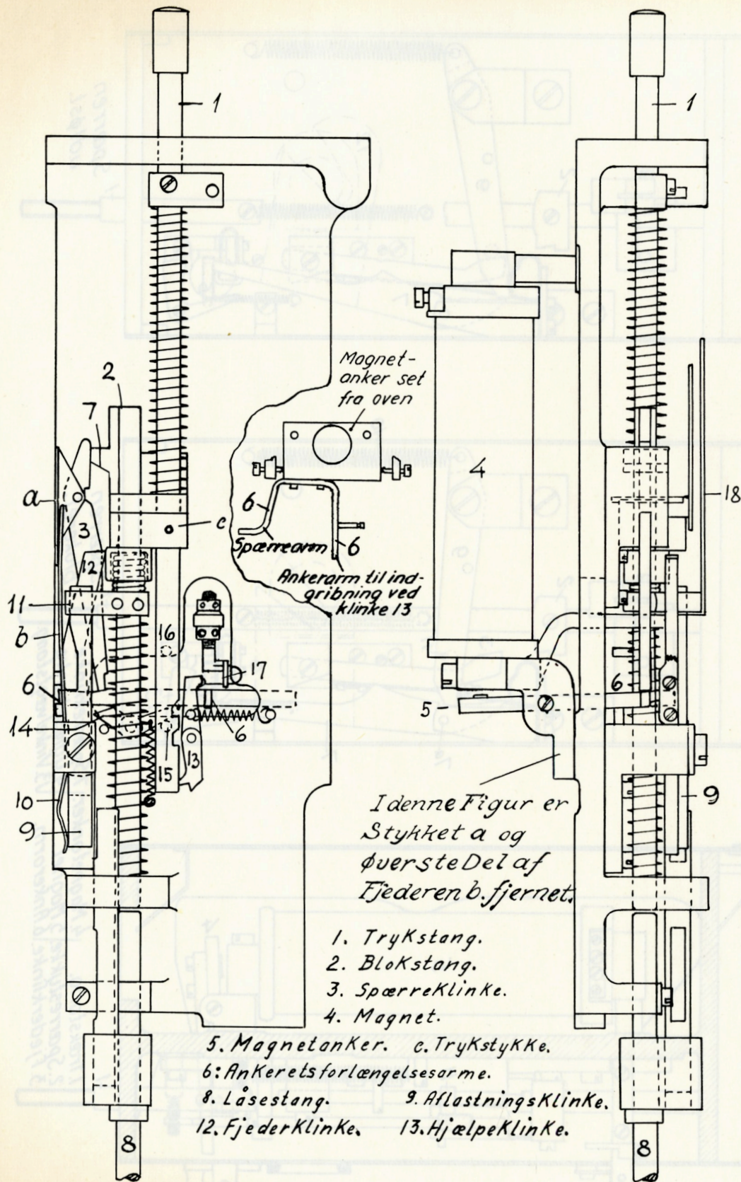
Fig. 0516b. Jævnstrømsblokfelt. (Siemens & Halske).
