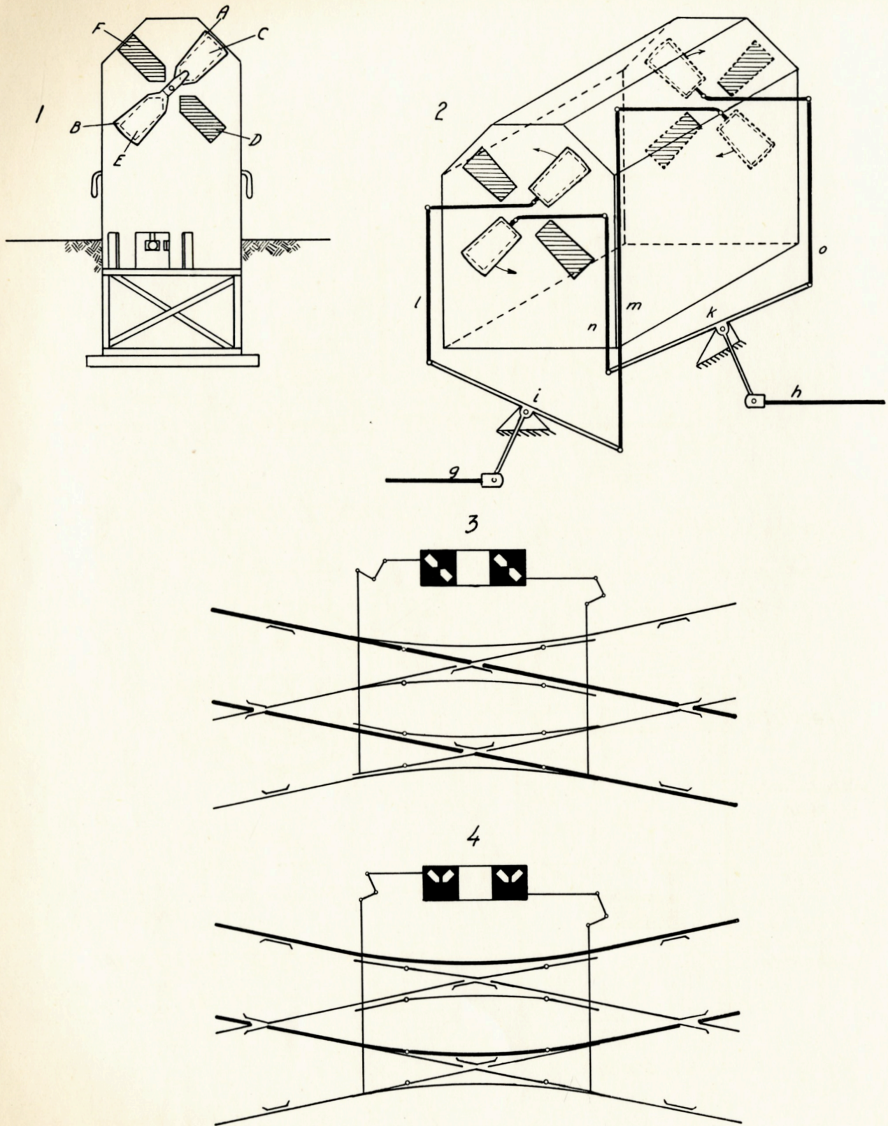
Fig. 0322. Vingelygte ved krydsningssporskifte.
