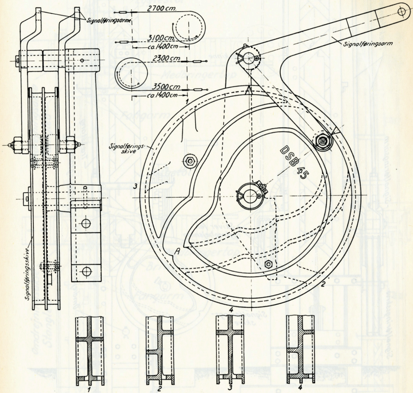
Fig. 0306. Mekanisk signaldrev D. S. B. 45.
