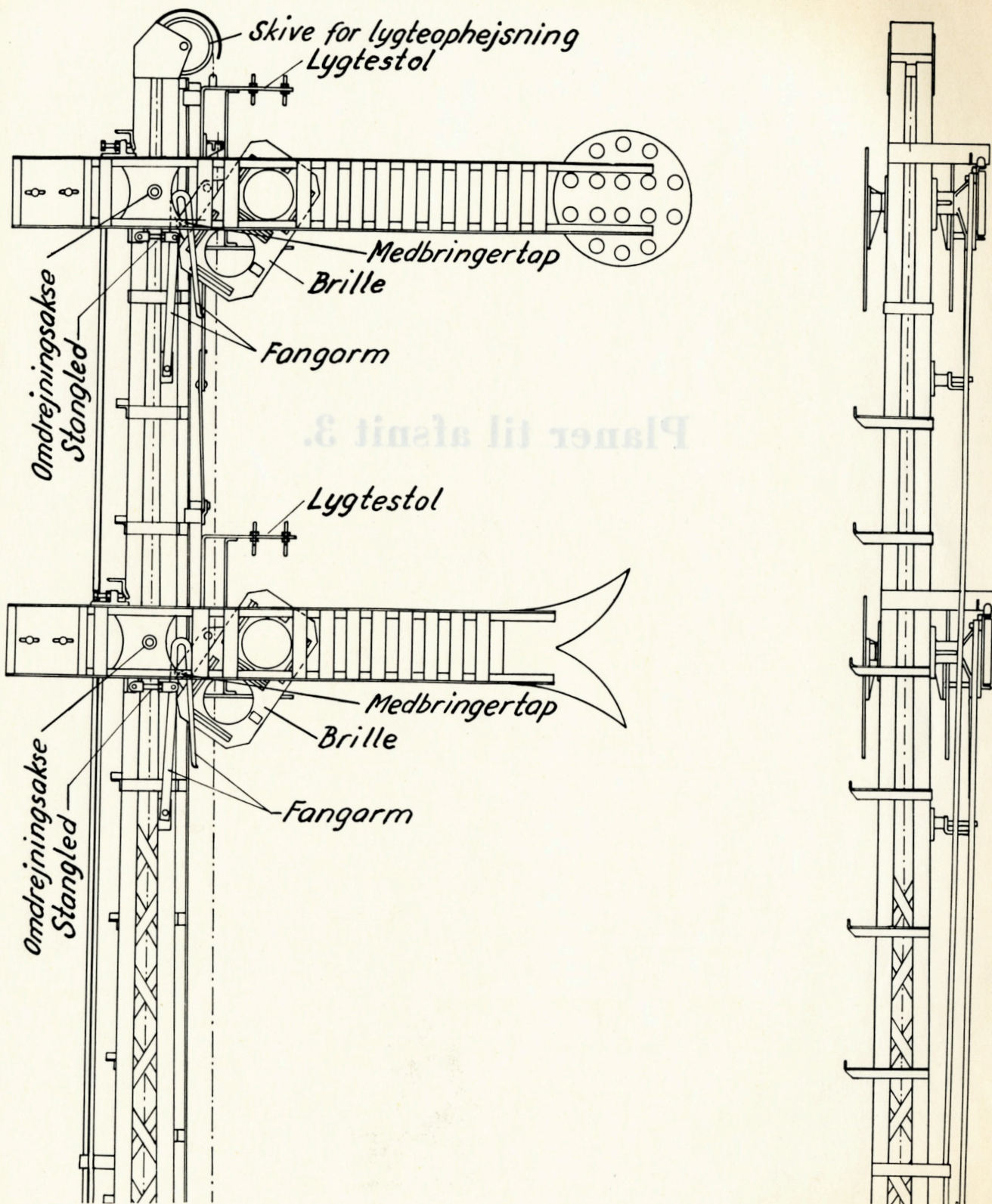
Fig. 0301. Øverste del af almindelig indkørselssignal med gennemkørselsarm.
