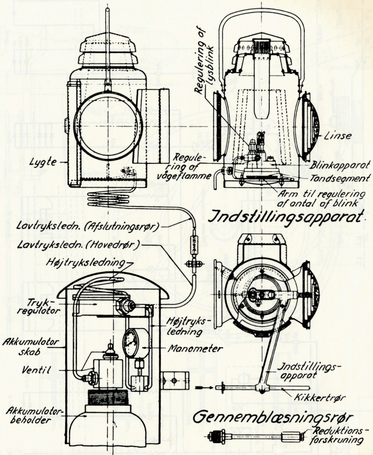
Fig. 0318. A. G. A. blinklysinstallation.
