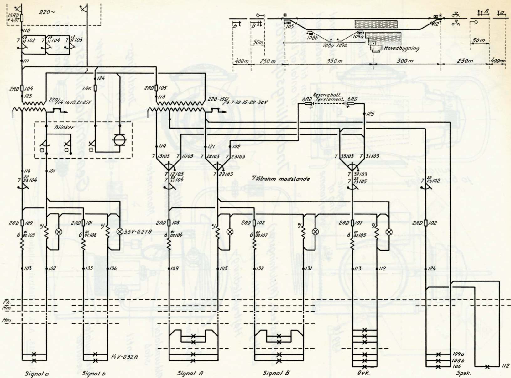
Fig. 0312. Strømplan for elektrisk signal-, sporskifte- og bombelysning på mindre station.
