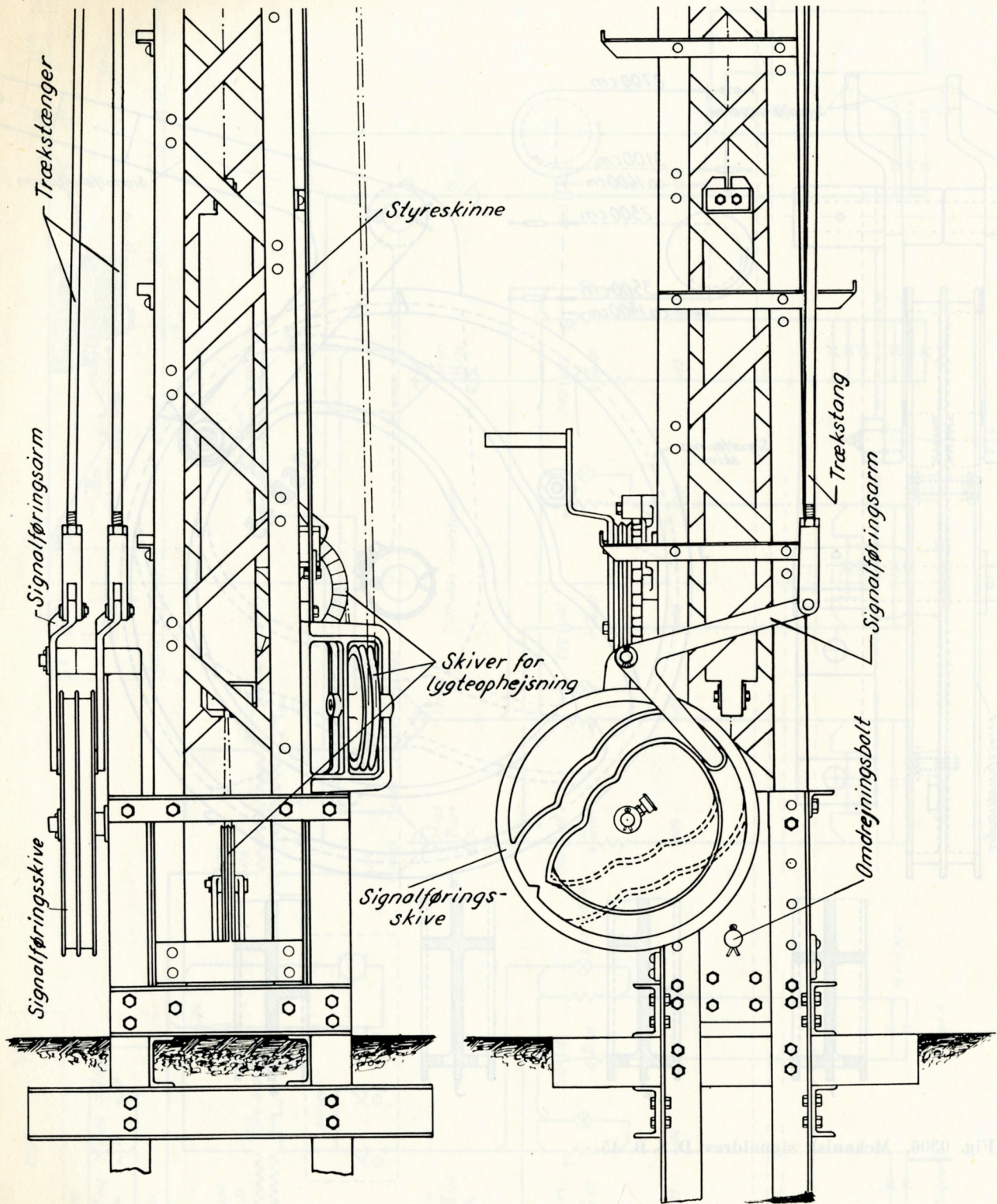
Fig. 0302. Nederste del af almindelig indkørselssignal med signaldrev m. v.
