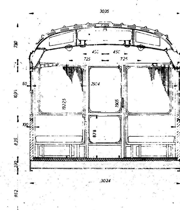
Snit A-A
